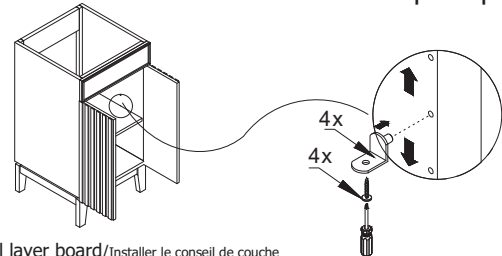
1. Install layer board/Installer le conseil de couche
